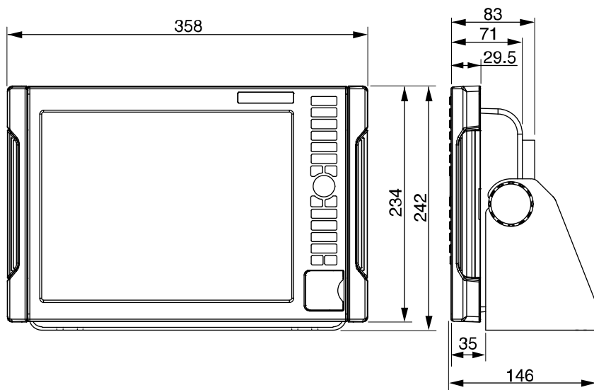
＜本体寸法図＞
